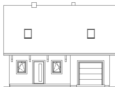
ELEWACJA FRONTOWA
