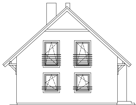
ELEWACJA LEWA
